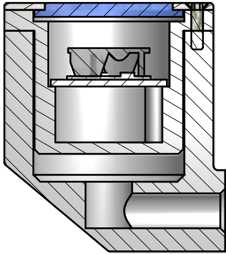
A-A ( .6 )
